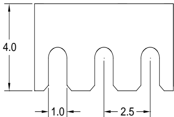
TYPE A (FEED-THRU)
