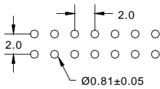
RECOMMEND P.C.B LAYOUT
