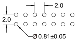
RECOMMEND P.C.B LAYOUT
