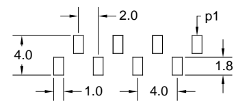
RECOMMEND P.C.B LAYOUT
