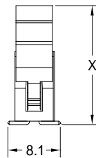
EJECTOR LATCH CAP (AVAILABLE)
